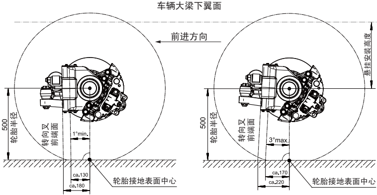
图5. 主销倾角
