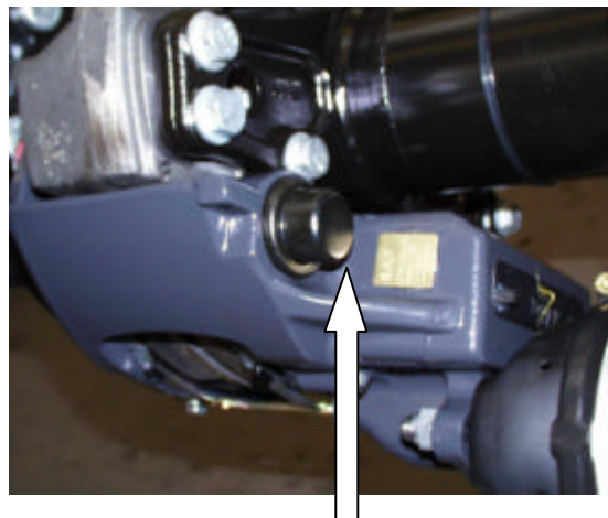
Bremse „neu“ mit Stahlkappe „new brake with steel cap
