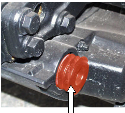
Bremse „alt“ mit Faltenbalg „old“ brake with rubber boot
